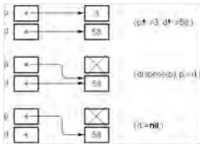
Рис. 13.2. Использование процедуры dispose
